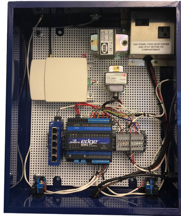
JENEsys® Edge™ 534
